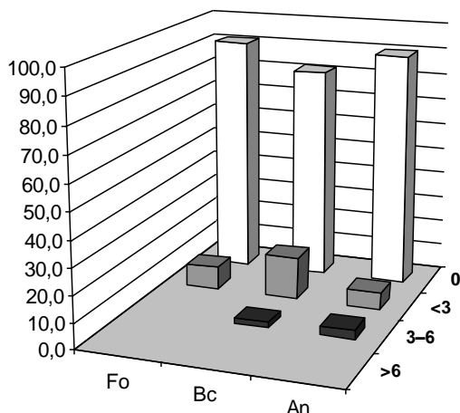
Рис. Антибактерійна (зліва) та антифунгальна (справа) активність штамів актиноміцетів із ризосфери T. roegneri K. Koch aggr. За віссю абсцис – ІА. За віссю ординат – кількість ізолятів, %. Ps – P. syringae , Pf – P. fluorescens , Psp – P. savastanoi pv. phaseolicola , Xcc – X. campestris pv. campestris , At – A. tumifaciens , Ea – E. amylovora , Fo – F. oxysporum , Bo – B. cinerea , An – A. niger .
